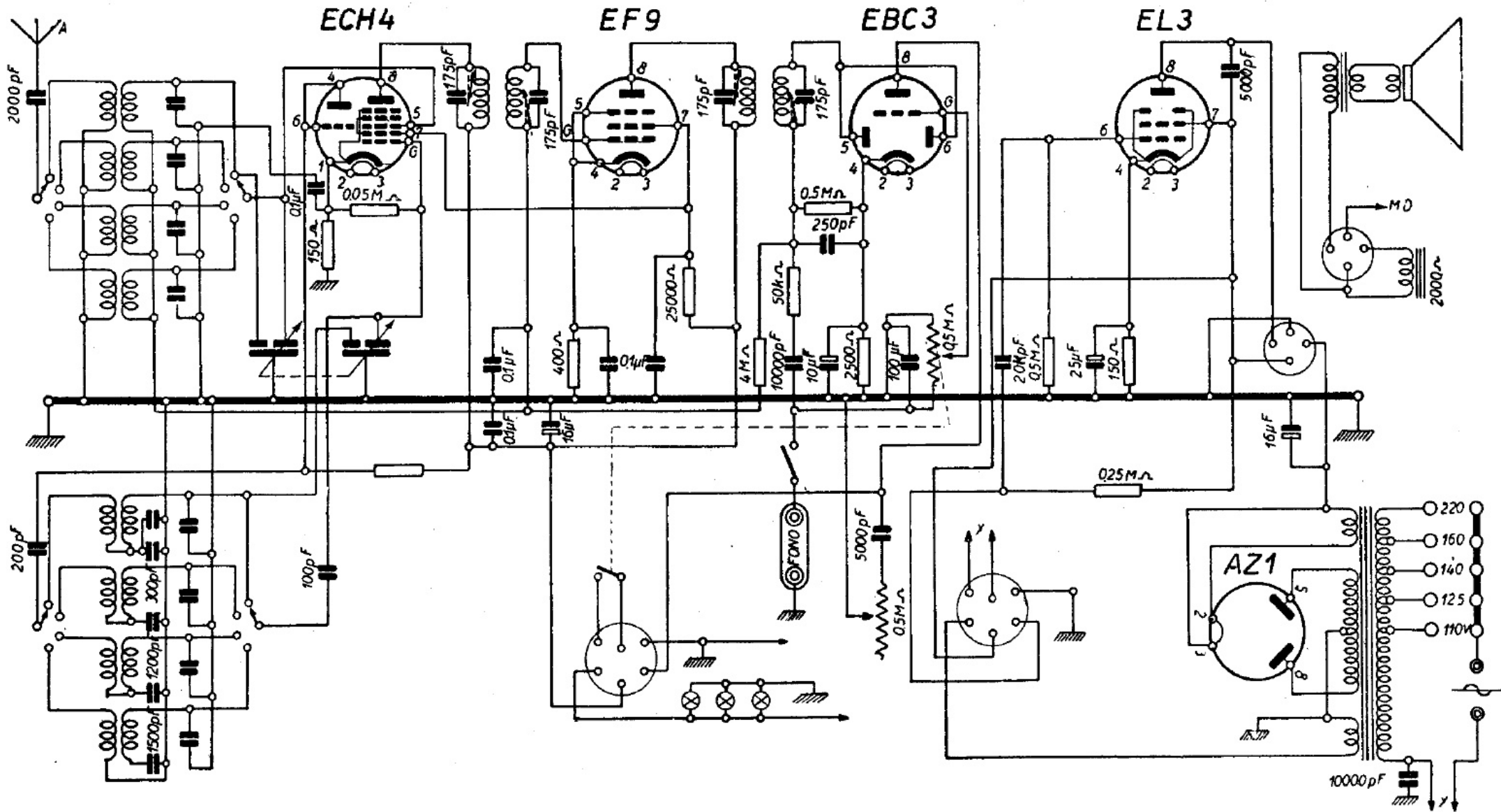
OREM (OFF. RADIO-ELETTROMECCANICA) - Mod. 542/R e Mod. 641 (con EM4 in più) - Il mod. 543 differisce dal mod. 542/R per avere la 6V6 G al posto della EL3. Il mod. 542 differisce dal 542/R per avere le seguenti valvole: 6A8 G, 6K7 G, 6Q7 G, 6V6 G e 5Y3 G). Il mod. 641 è identico al mod. 542 con la EM4 in più. Media frequenza 467 kc/s.
